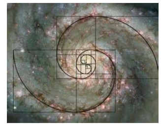
Vía Láctea.
